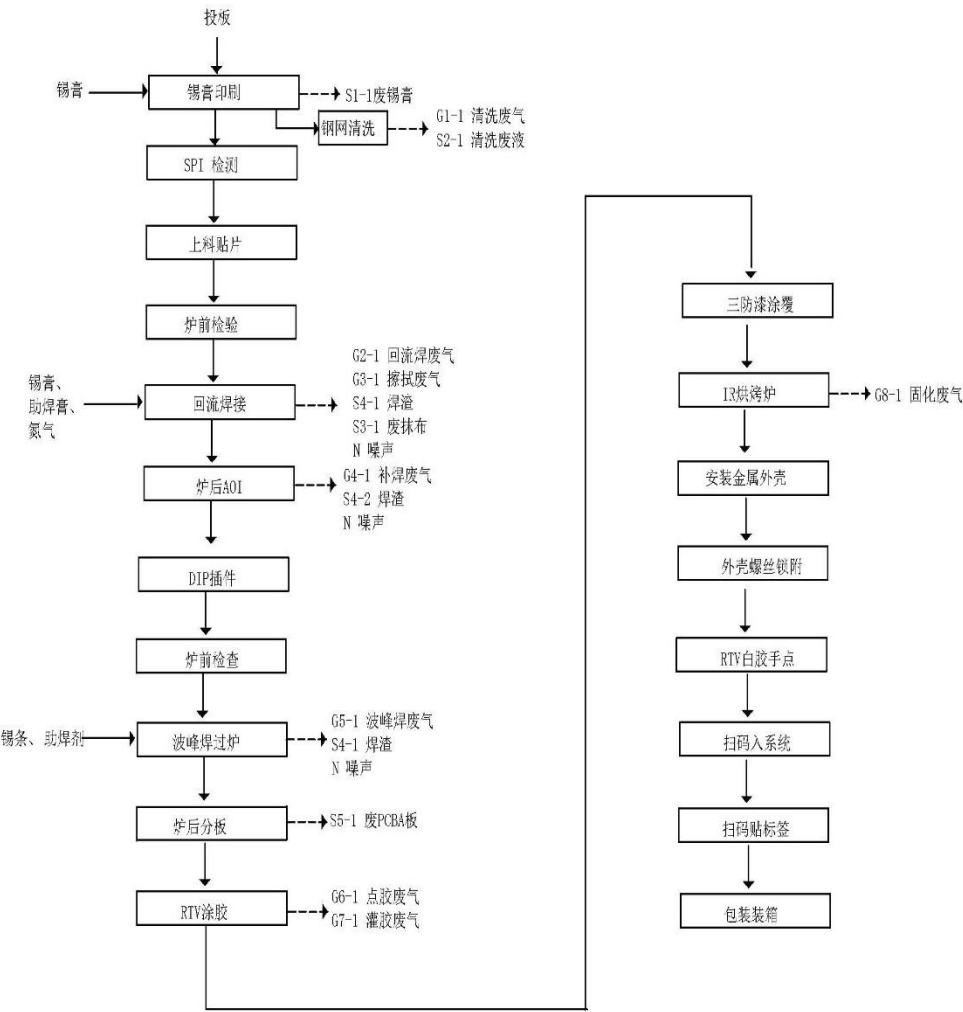
图 2-3 本项目产品生产工艺流程图
