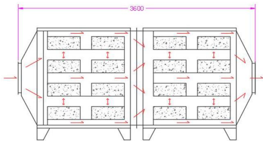
图 4-1 活性炭箱结构图
