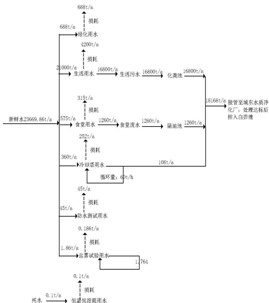
图 2-1 扩建后全厂水量平衡图
